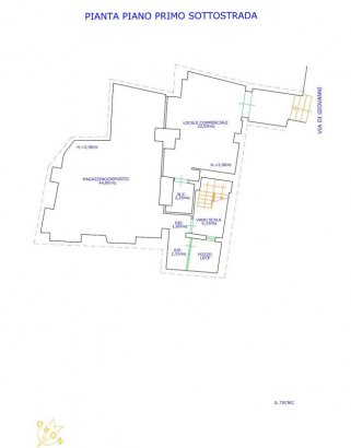
PLANIMETRIA DEI LOCALI Scala 1:100 - "STATO DI FATTO"
